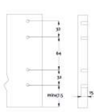
dimensões de perfuração do painel frontal
