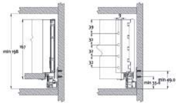
espaço necessário no armário Dimensões de instalação do painel traseiro
