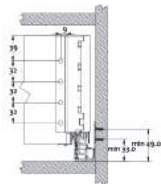
dimensões de instalação do painel traseiro
