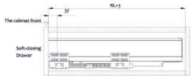
dimensões da cabine p/gaveta
