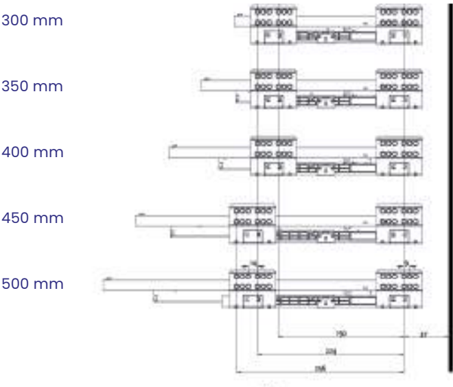
dimensões da cabine p/gaveta
