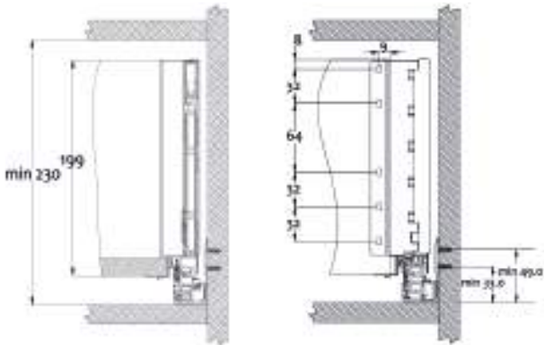
espaço necessário no armário Dimensões de instalação do painel traseiro
