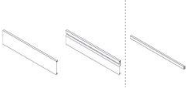
REF. 0486 painel sem puxador REF. 04H86 painel com puxador REF. 0-05 vareta quadrada
