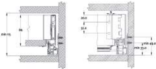
dimensões da cabine p/gaveta
